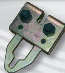
SP706320 STAFFA LARGA DI TIRO 2 DIREZIONI 5T (RETTO) 3T (VERTICALE) / 5T (STRAIGHT) 3T (VERTICAL) DOUBLE DIRECTION LARGE PULLING CLAMP
